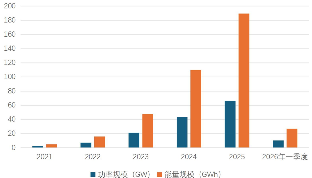
图表 19: 国内新型储能新增装机规模 (GW, %)
